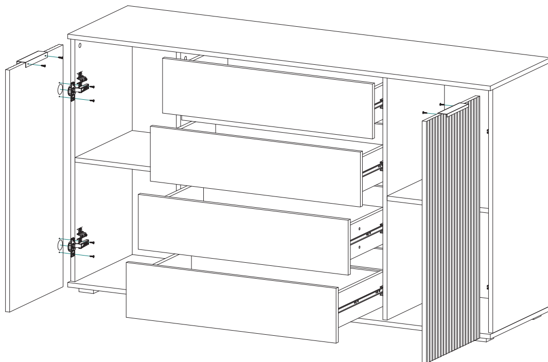
схема монтажа петли
