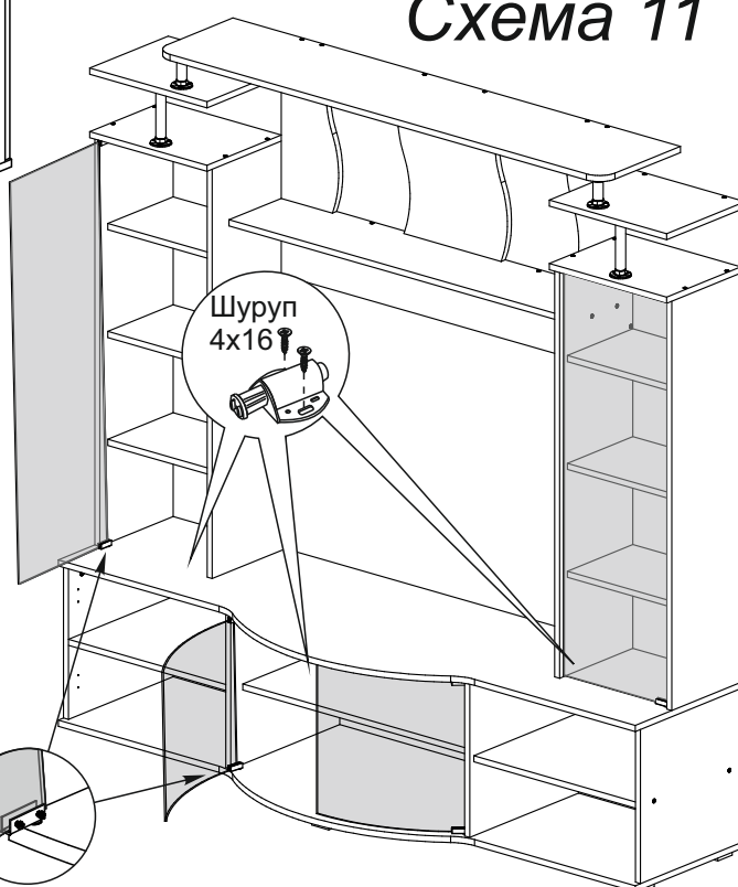
Схема установки стекловорки №26 и №27 в стеклопетлю
